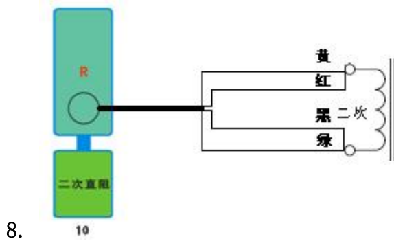
7. 接线图：图七（二次直阻接线图）
